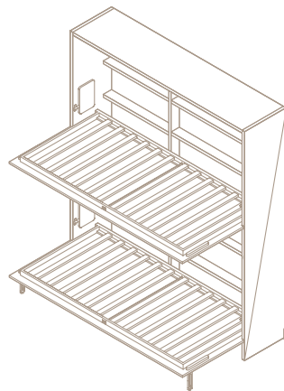
Cama doble Double bed
